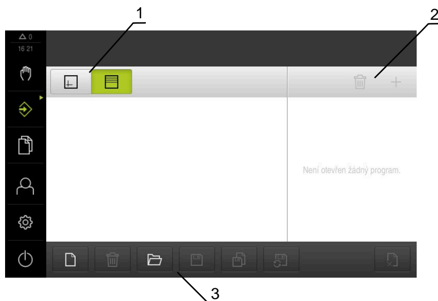
Obrázek 9: Menu Programování
